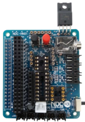
ロボットコントロールボード
