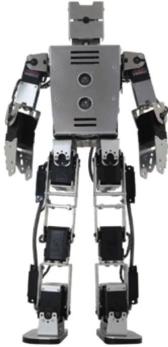
教育用人型ロボット「NDC-HN01」
